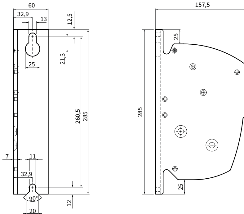
Vorderansicht Wandhalterung links
