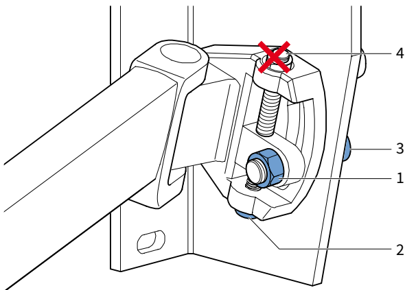
Abb. 4.1 Detail Armverbindung rechts
