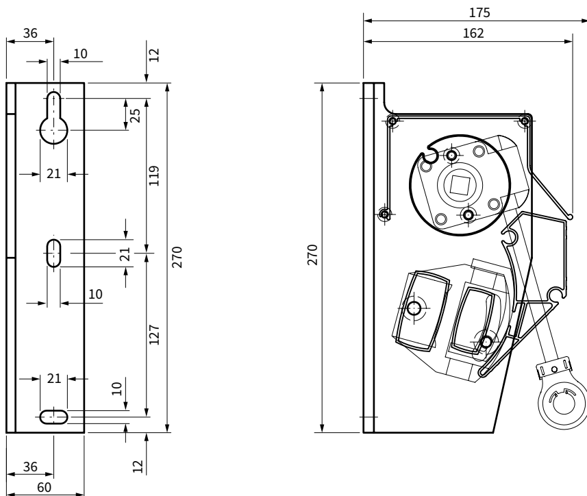
Vorderansicht Wandhalterung links
