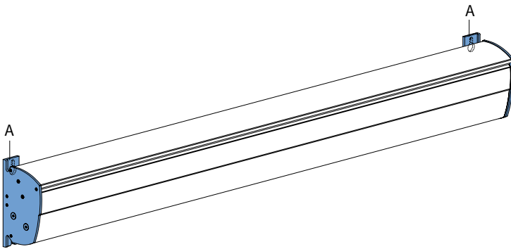
Abb. 1.1 Wandhalterungen Gelenkarm-Markise
