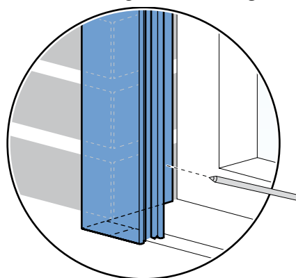
in der Laibung, LHTF Führung
