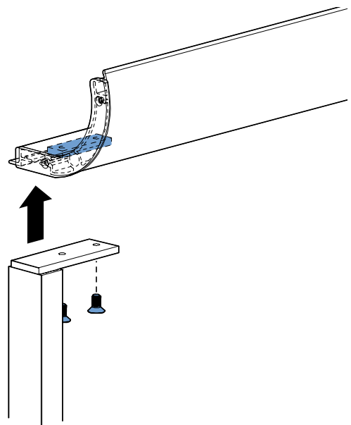
Abb. 3.8 Festschrauben des Ausfallarms
