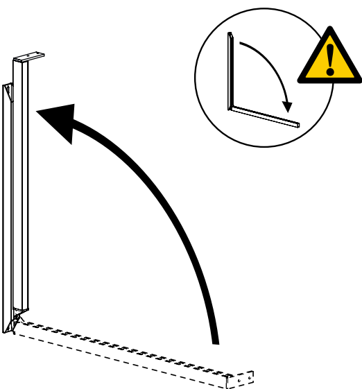
Abb. 3.7 Zurückklappen des Ausfallarms
