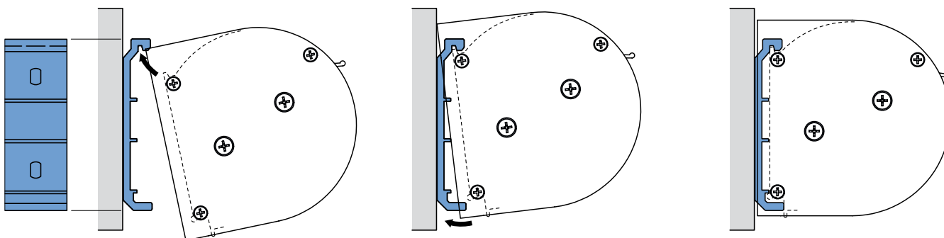
Abb. 2.2 Detail der Wandhalterung
