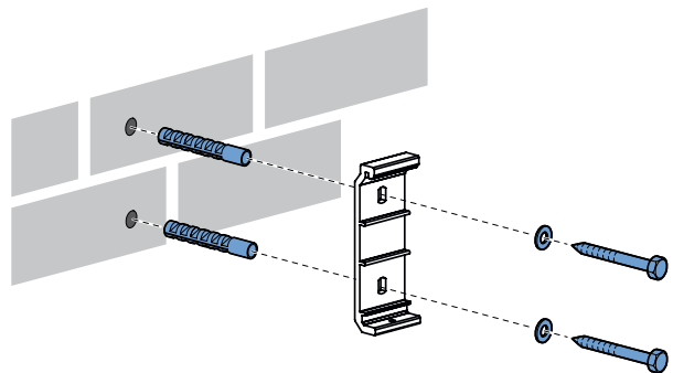
Abb. 1.3 Montage Wandhalterung
