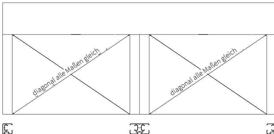
Abb. 6 Draufsicht
