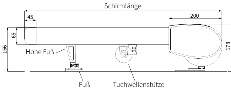
Abb. 1 Seitenansicht Abmessungen
