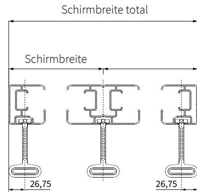
Abb. 2 Vorderansicht
