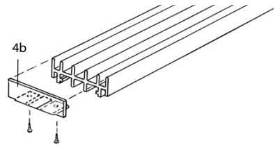
Abb. 2.2 Abschlusskappe der unteren Schiene
