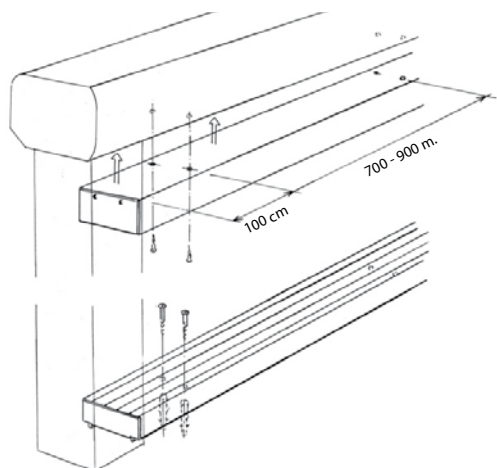
Abb. 3.2 Montage der oberen Abdeckung und der unteren Schiene
