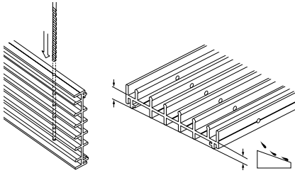
Abb. 1.1 Entwässerungsbohrungen in der unteren Schiene anbringen
