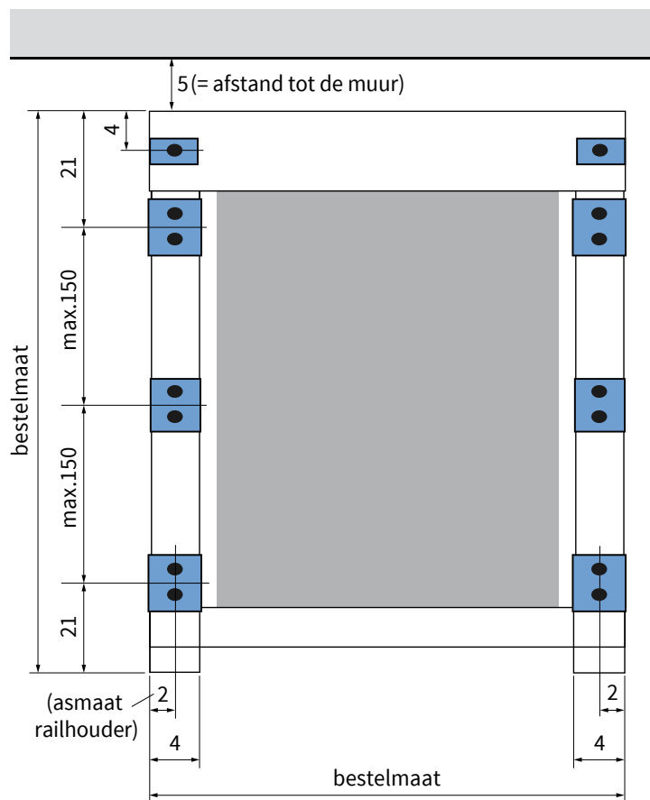
Fig. 1 Boven aanzicht verandazonwering
