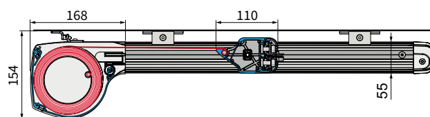
Fig. 3 Doorsnede verandazonwering
