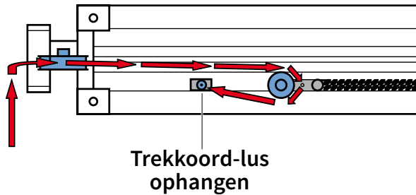
Koordverloop in het uitvalprofiel aan de linkerzijde
