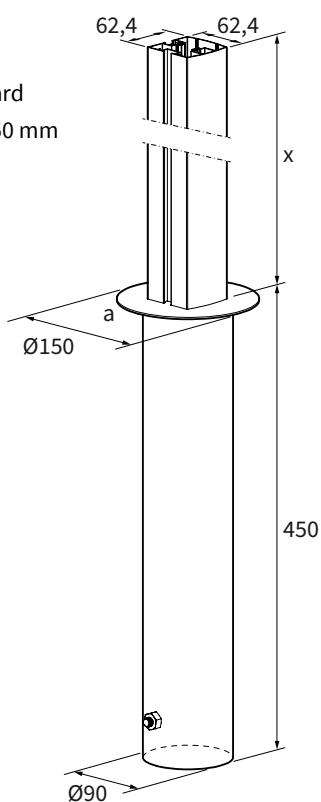
Hoekprofiel
