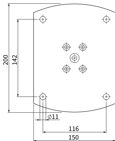
Grond voetplaat
