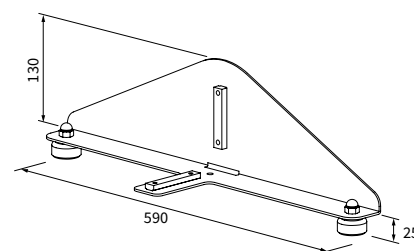
Verstevigde voet
