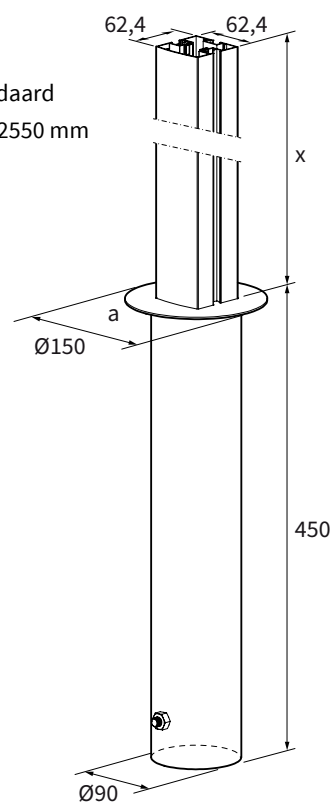
T-profiel
