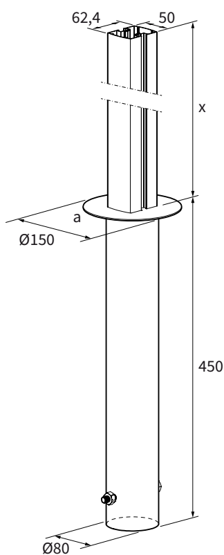
Tussenprofiel
