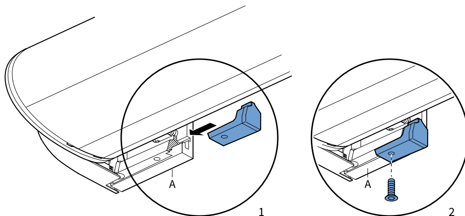
fig. 2.4 Detail borgblokje
