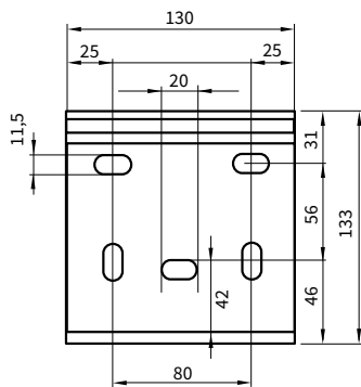
vooraanzicht muursteun
