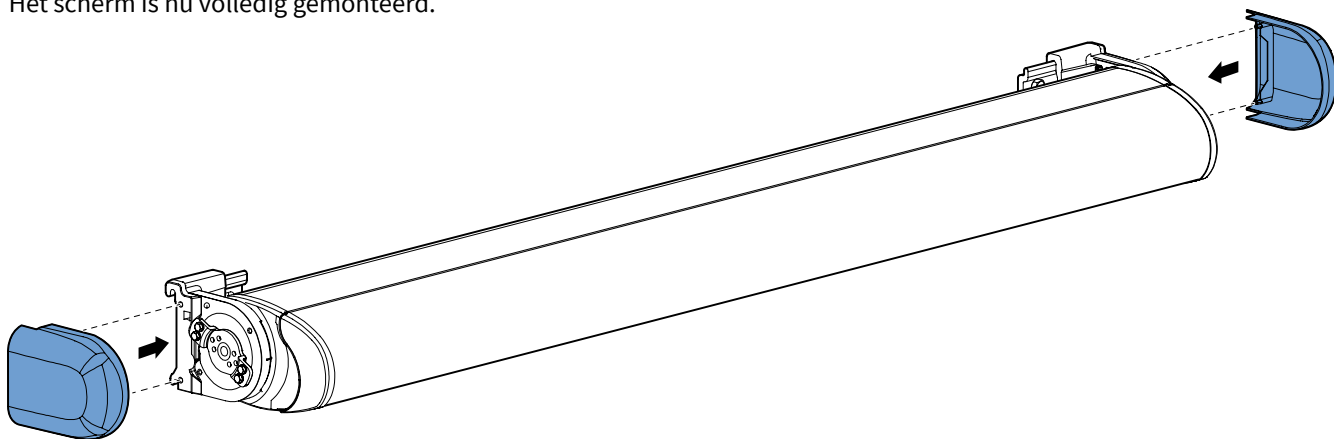
fig. 7.1 Monteren zijkappen
