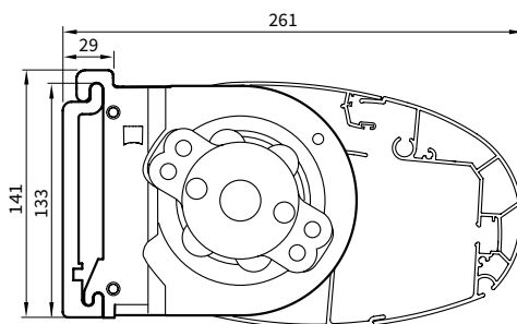
schermdoorsnede
