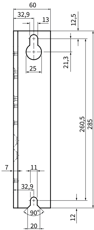
vooraanzicht muursteen links
