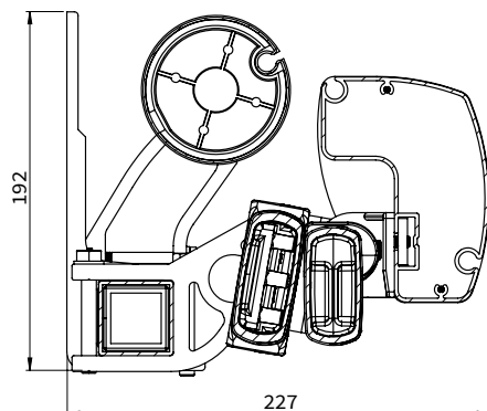
schermdoorsnede
