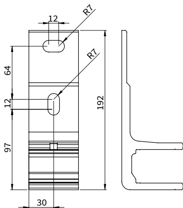
muursteun
