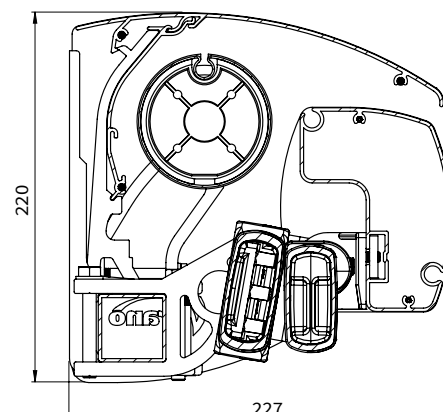
schermdoorsnede van uitvoering met omkasting
