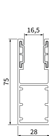
doorsnede UPH 240 geleider (G)
