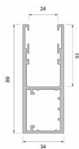
doorsnede UPH 89 geleider (G)
