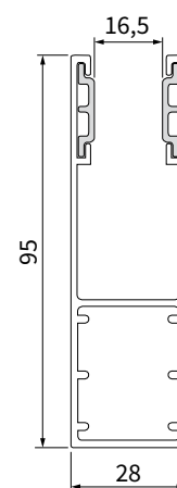
doorsnede UPH 260 geleider (G)
