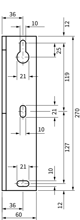
vooraanzicht muursteun links
