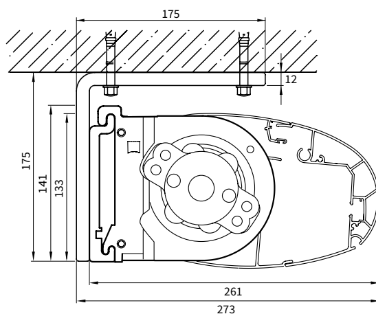
schermdoorsnede
