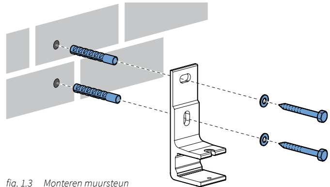
fig. 1.3 Monteren muursteun
