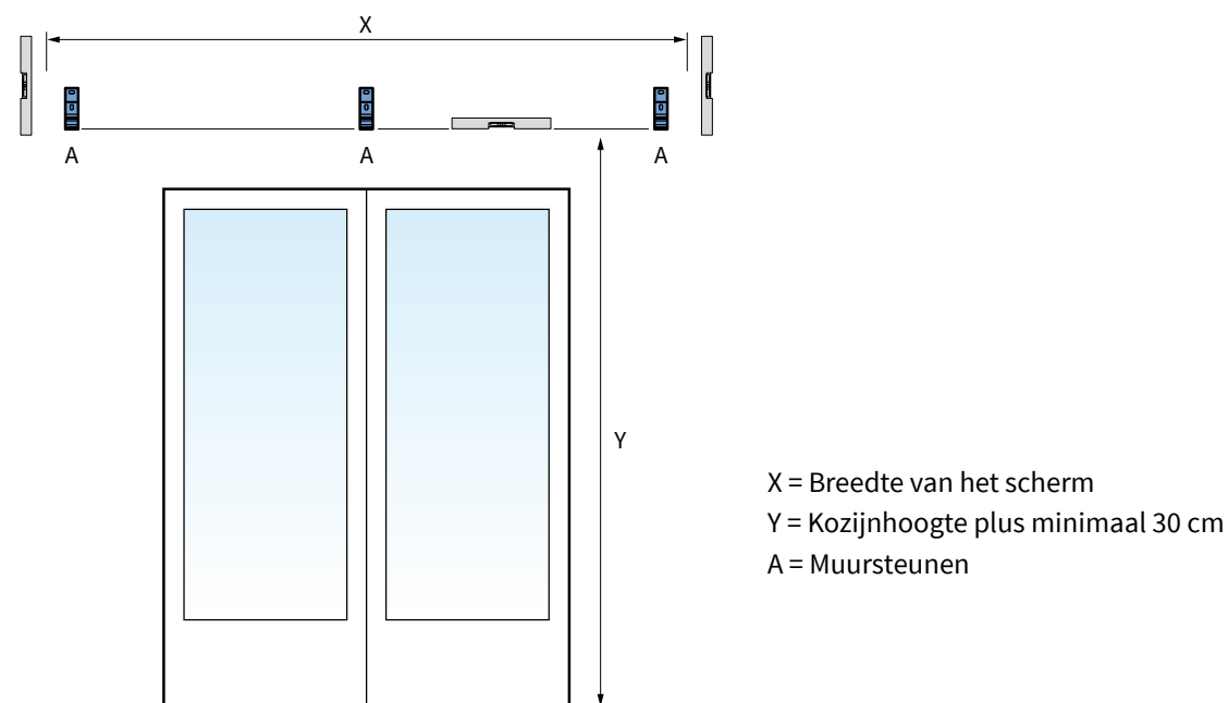
fig. 1.2 Plaatsing muursteunen
