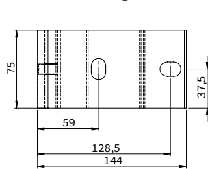
vooraanzicht muursteun
