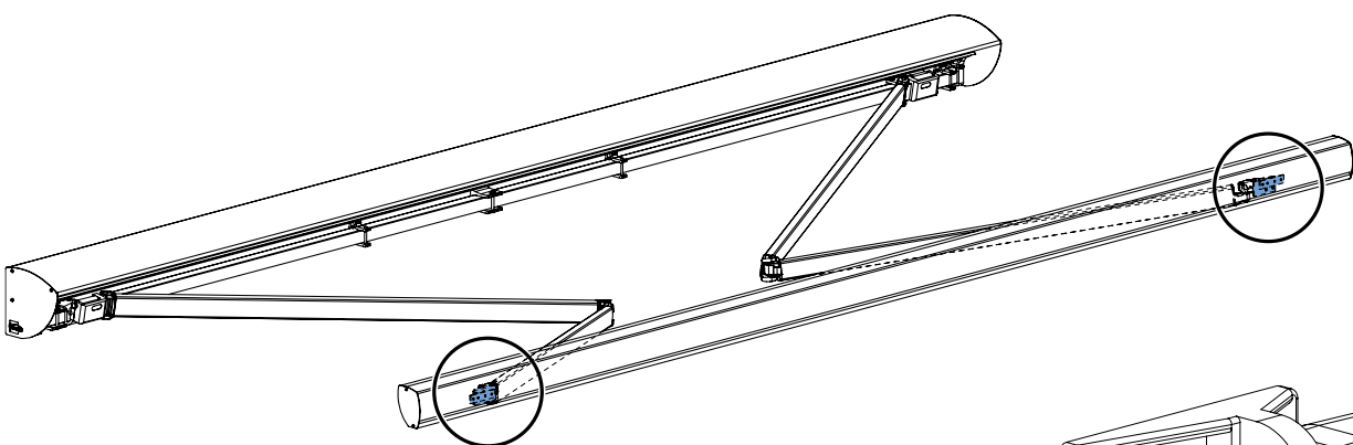
fig. 6.2 Locatie armverbindingen
