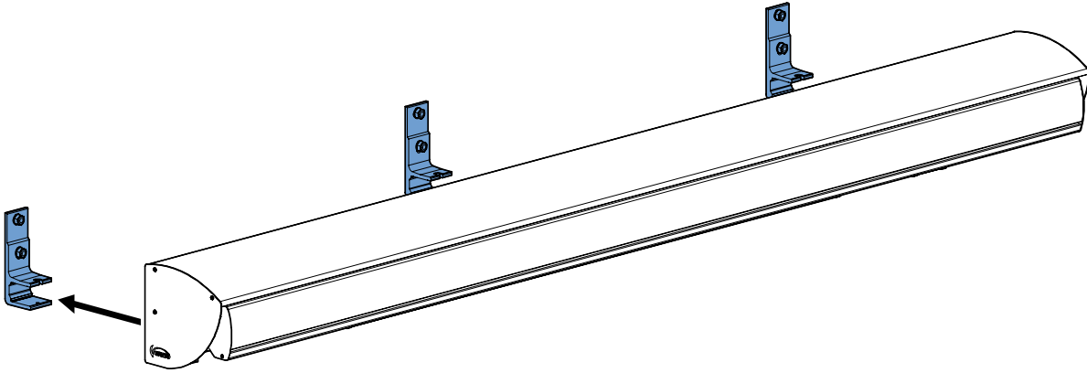
fig. 2.1 Ophangen scherm
