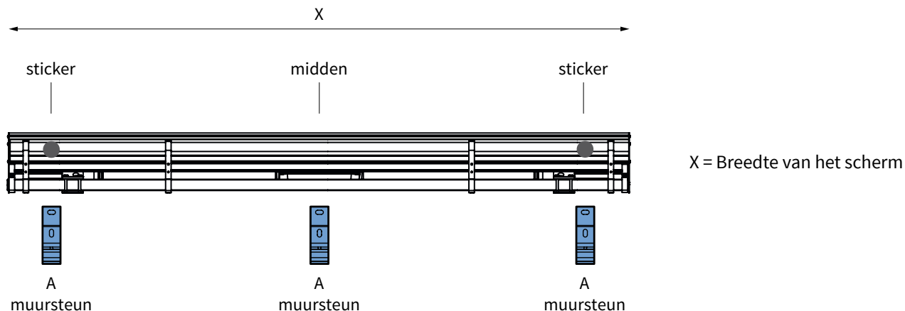
fig. 1.1 Plaats stickers
