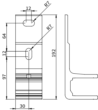
vooraanzicht muursteun
