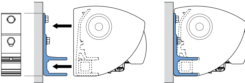
fig. 2.2 Detail muursteun
