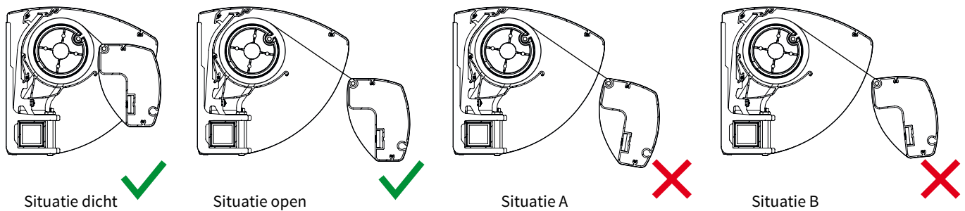
fig. 6.1 Positie voorlijst
