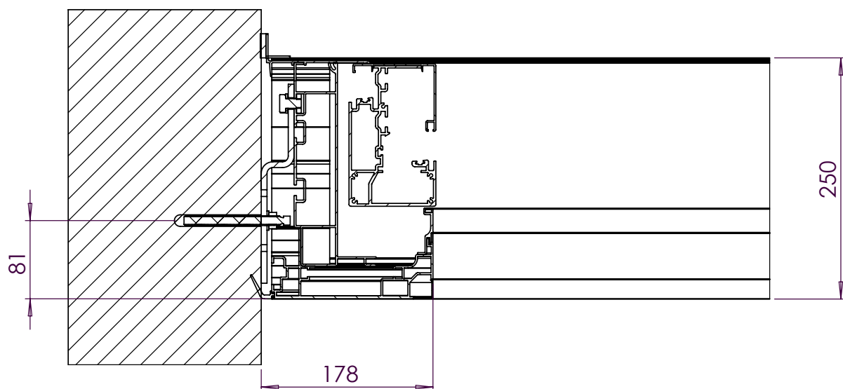
SECTION A-A SCALE 1 : 5
