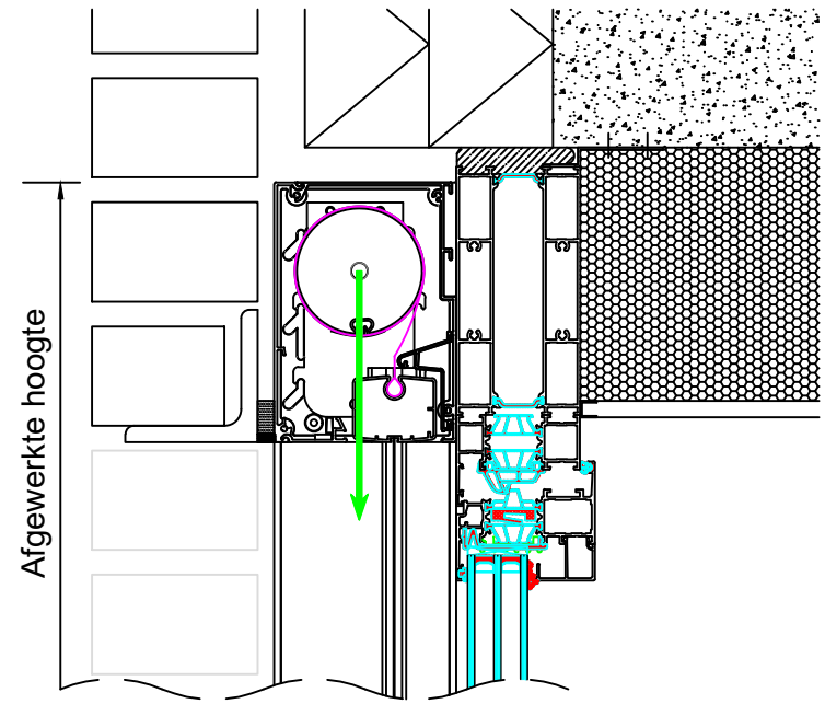
Metselwerk
