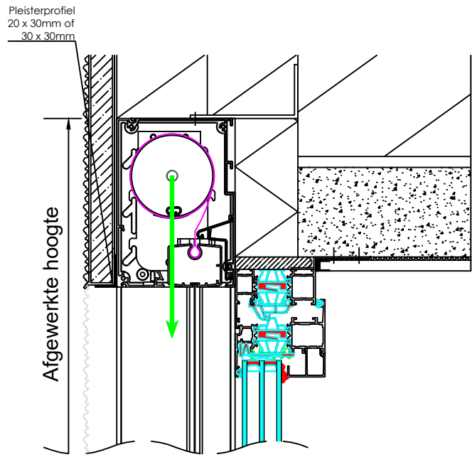
Pleisterwerk
